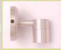
GL-172/S / Arbotante Simple MR-16 Satinado Medidas: Ø 14.0 cm x H15.3cm Foco: MR-16 / WT: 50 Volts: 12
